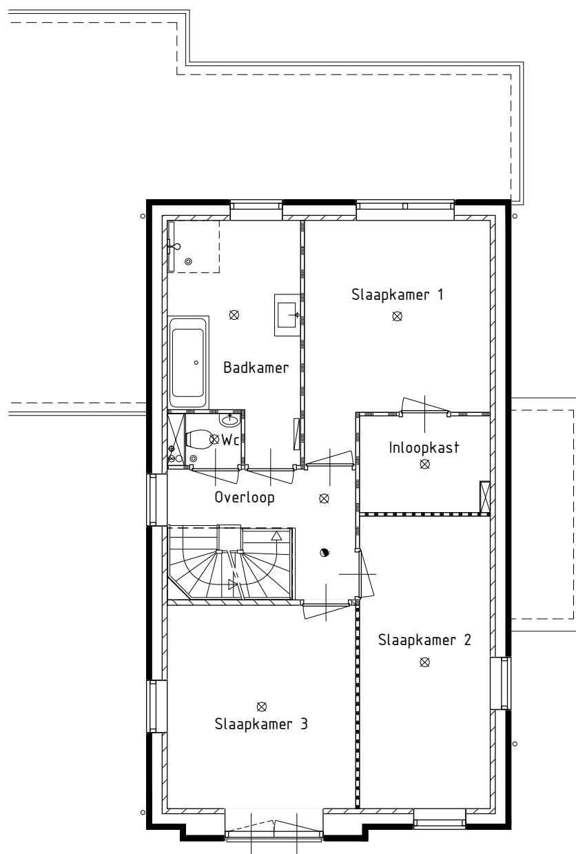
1ste Verdieping
