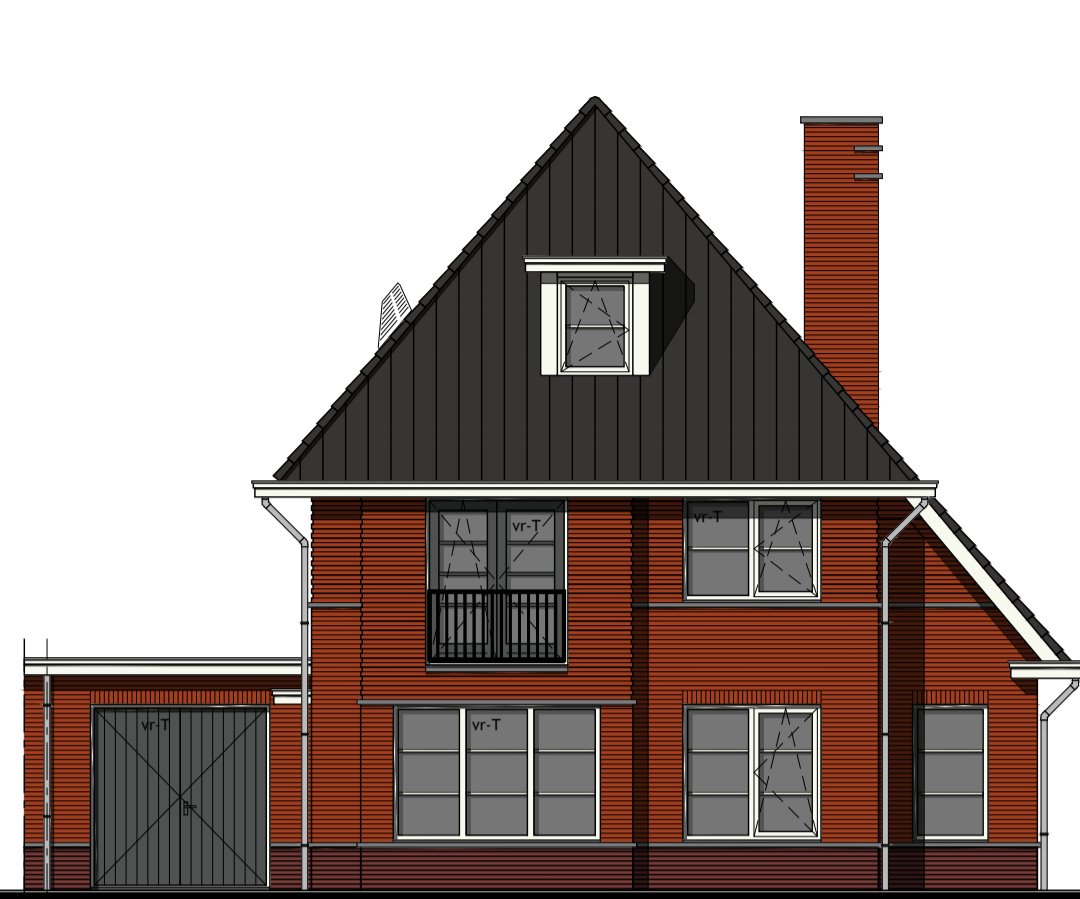
Voorgevel
