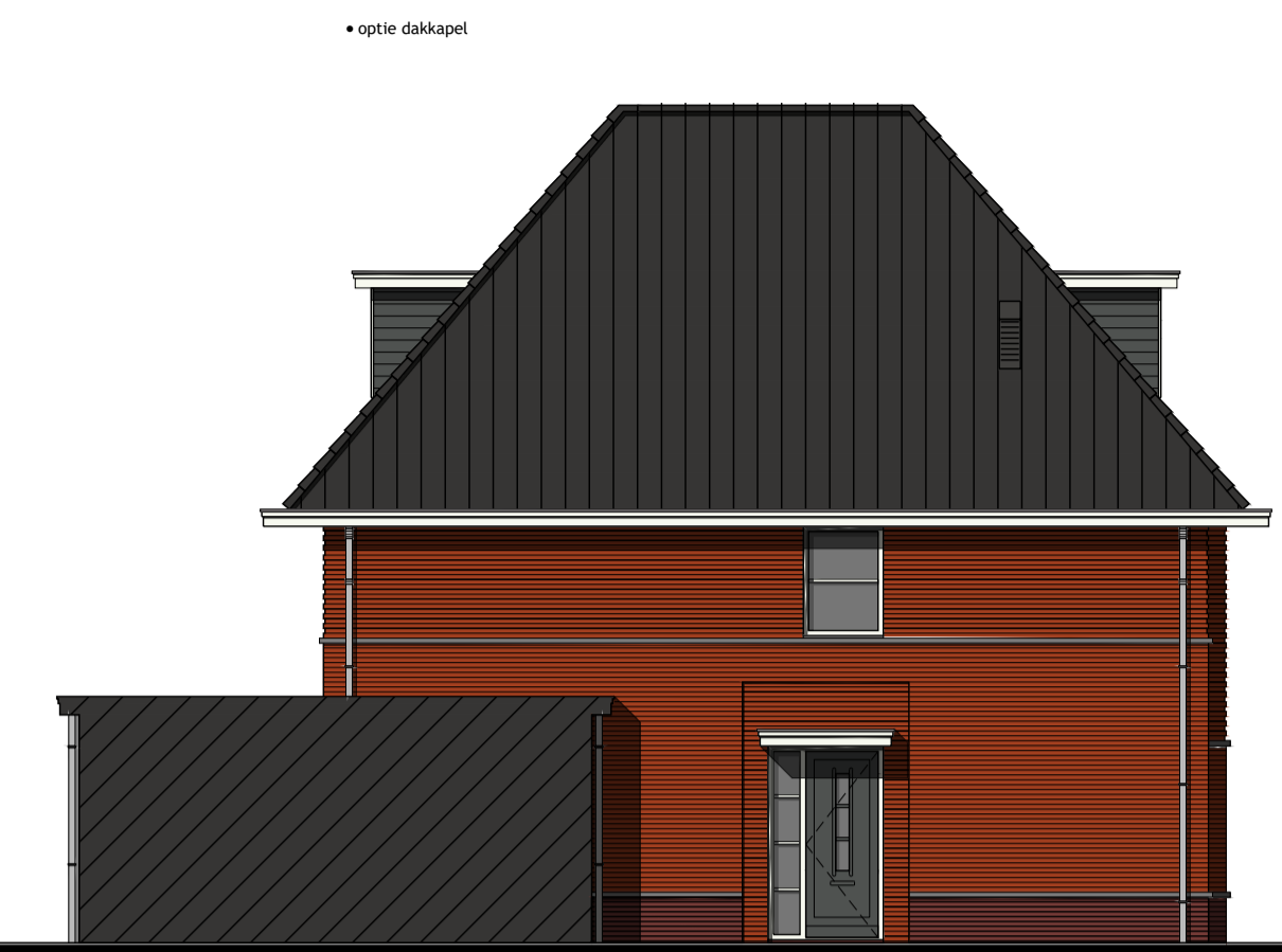
Linker zijgevel
