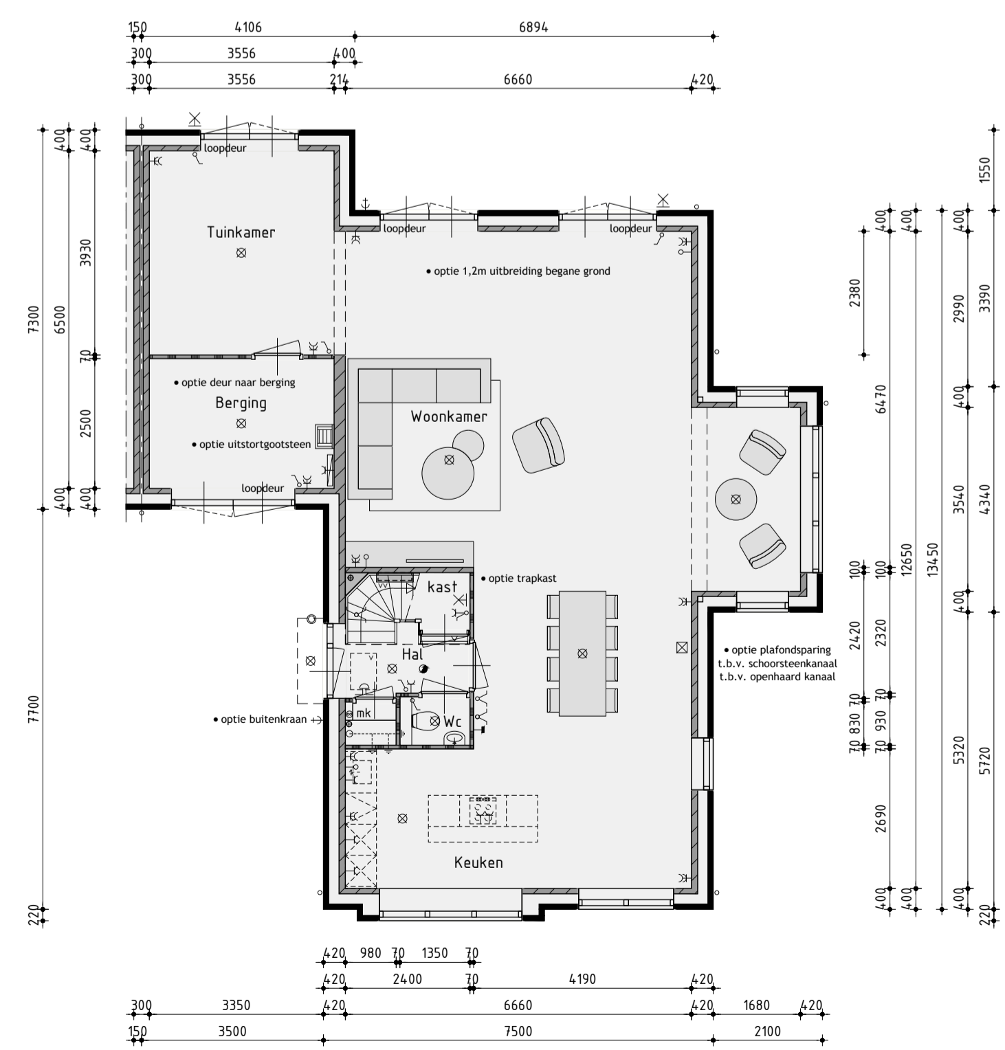
Begane grond v.z.v. vloerverwarming
