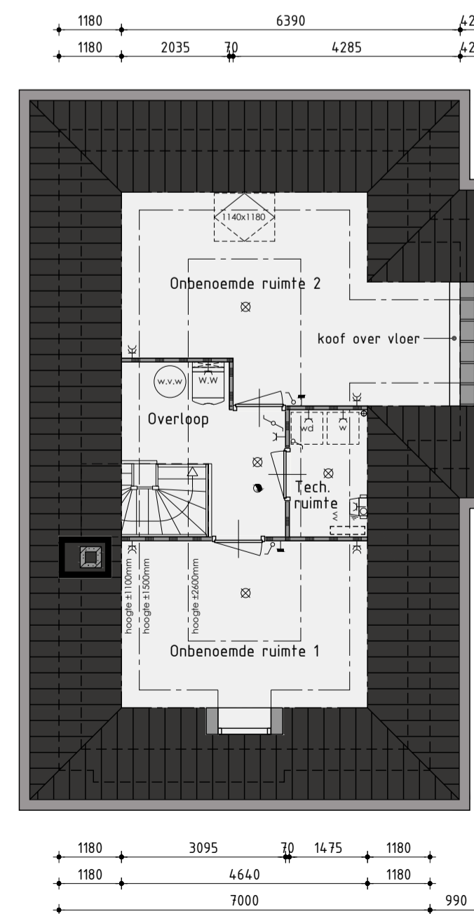
2de Verdieping
