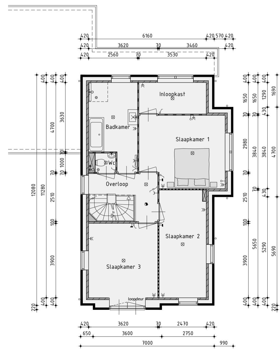
1ste Verdieping
