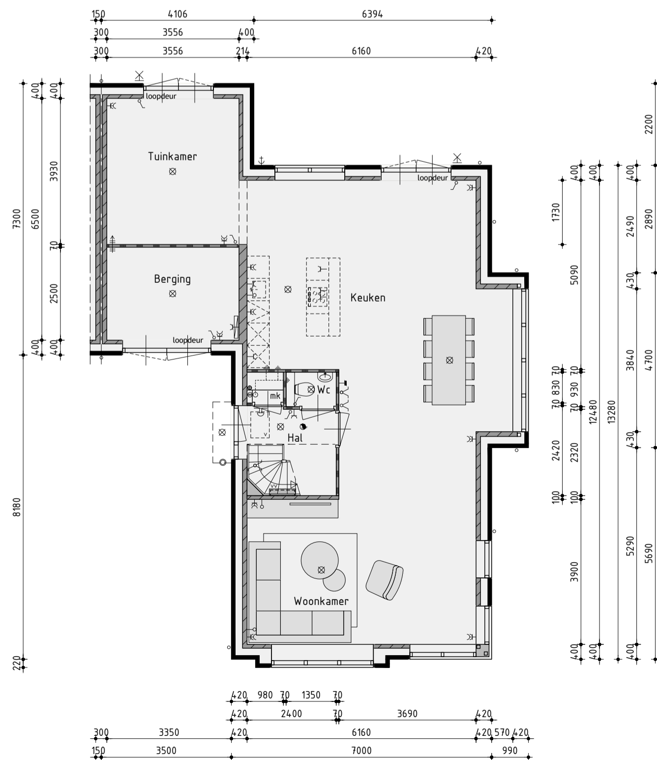
Begane grond
